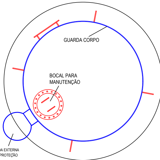
VISTA SUPERIOR sem escala
