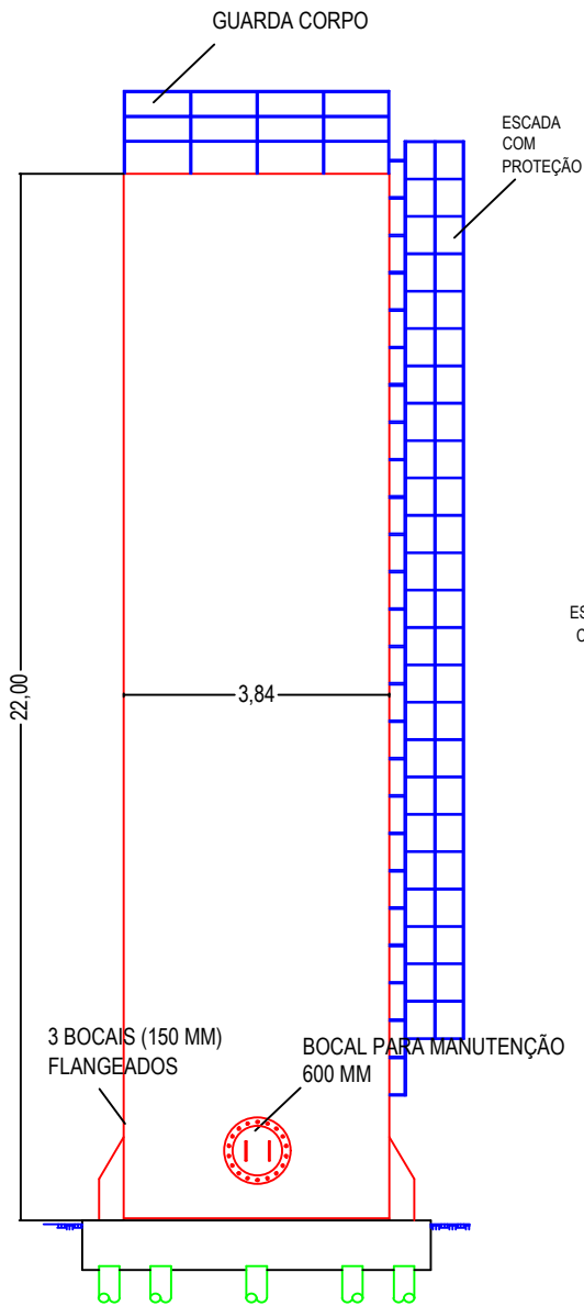
VISTA FRONTAL sem escala
